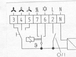
Kapcsolási rajz (KLR-E 7203):
